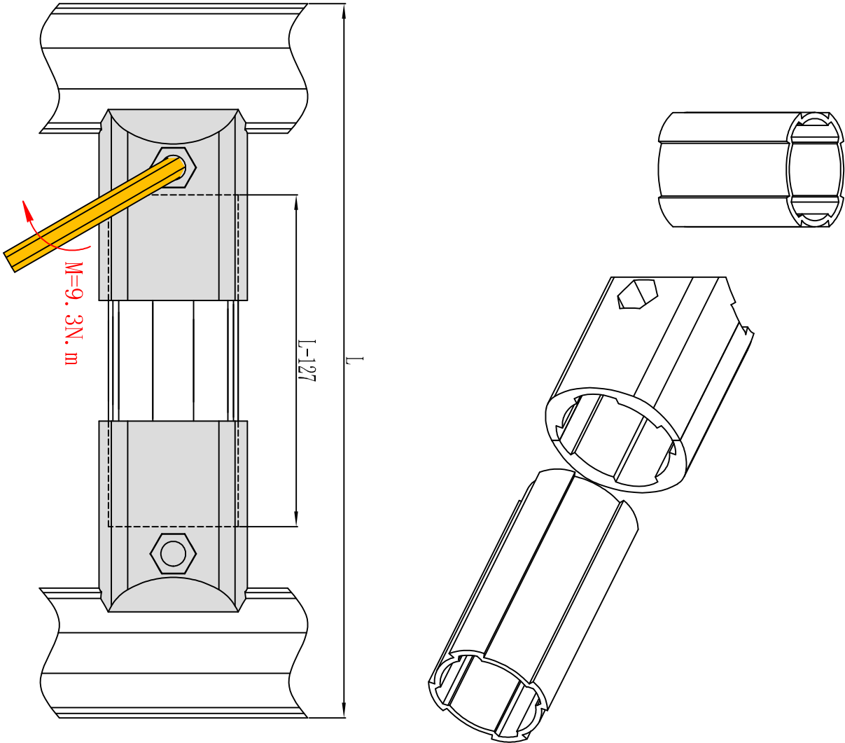
安装示意图
